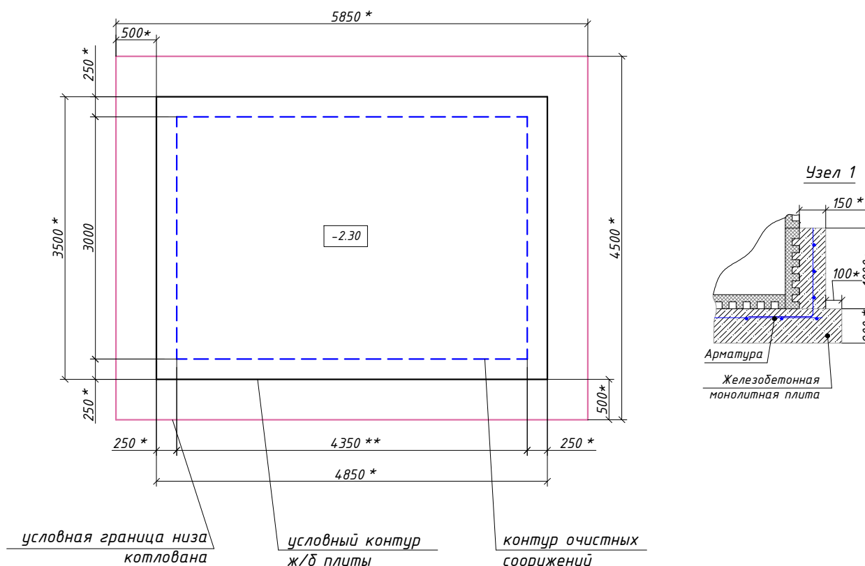
План котлована с плитой
