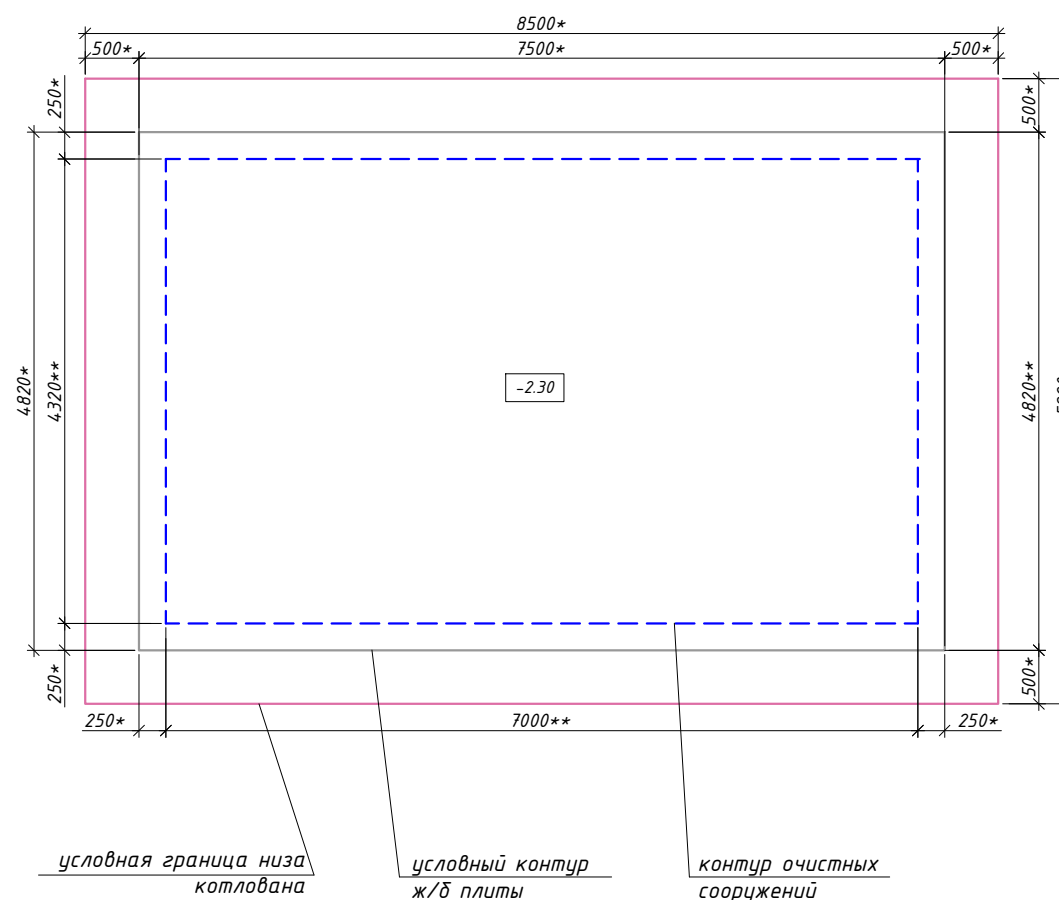
План котлована с плитой
