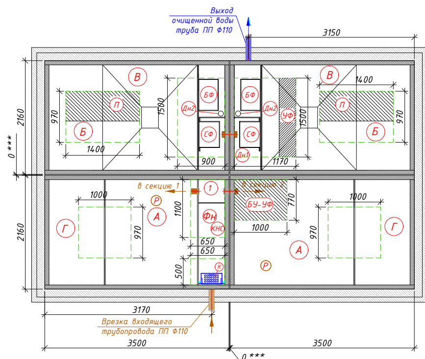
Схема станции
