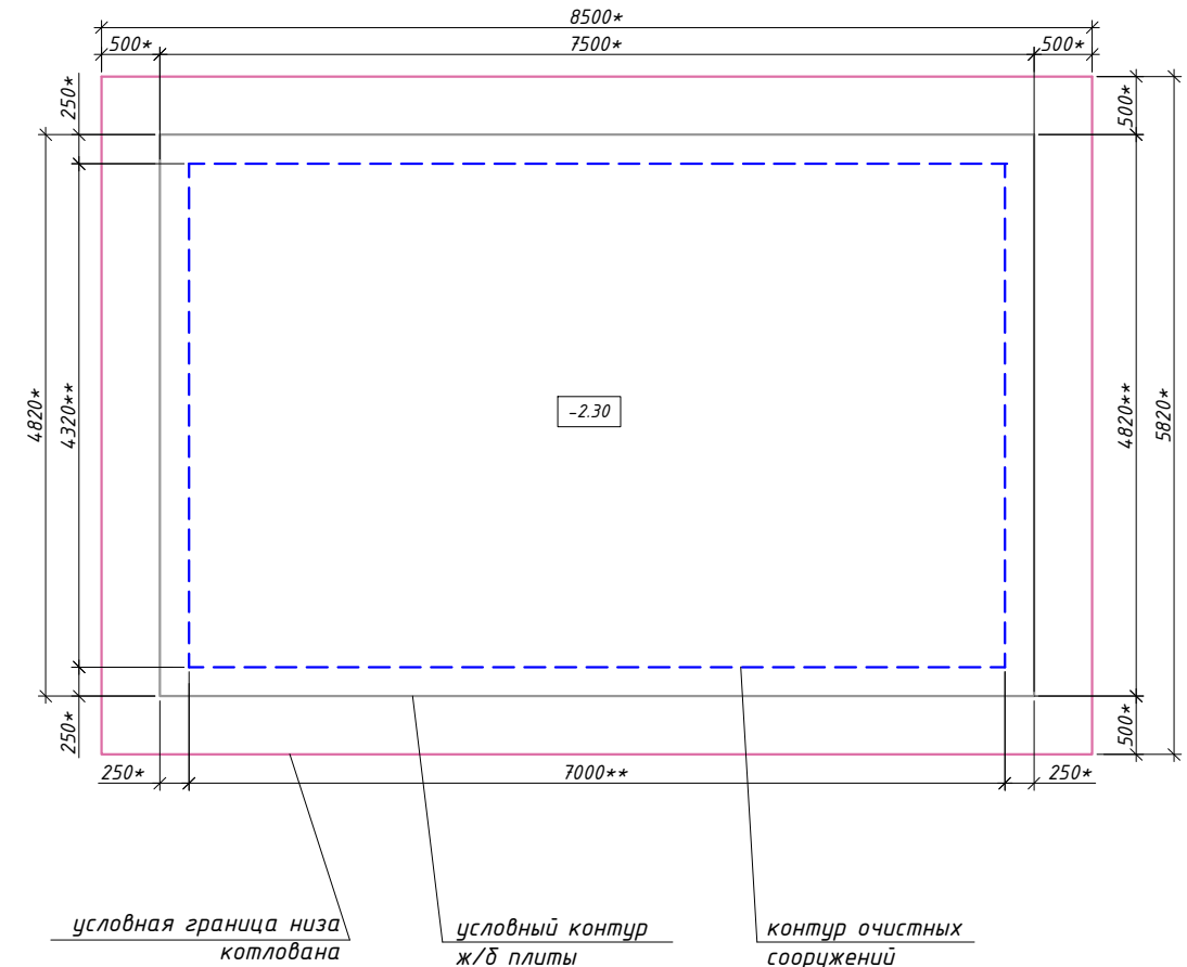
План котлована с плитой
