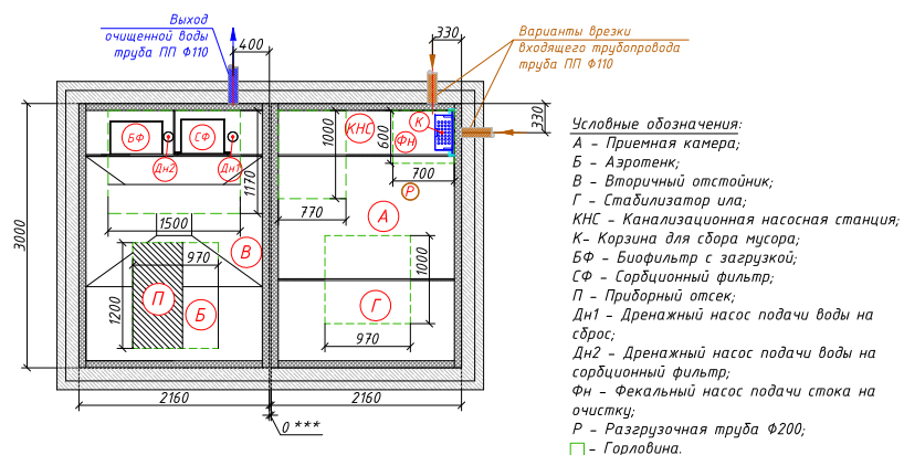
Схема станции
