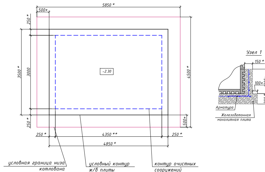
План котлована с плитой
