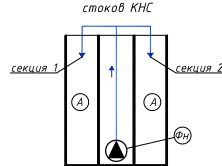
Схема распределения стоков КНС
