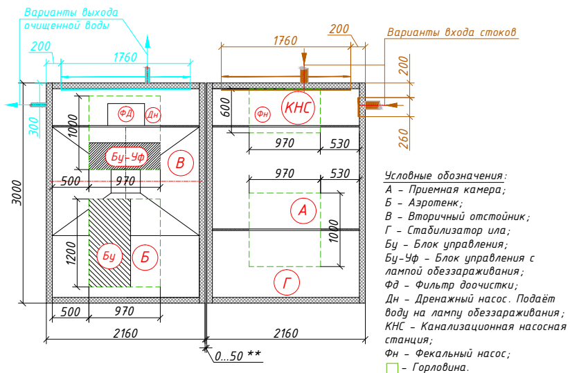
Схема станции
